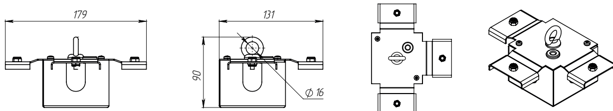
ДСО_кронштейн_15_СБ
