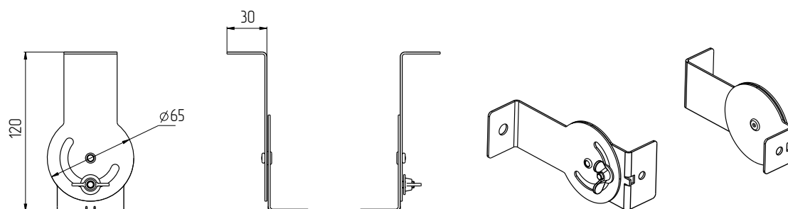
ДСО_кронштейн_109_СБ
