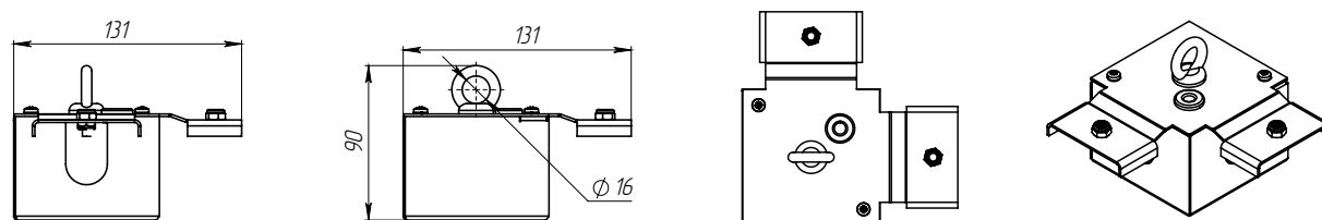
ДСО_кронштейн_16_СБ
