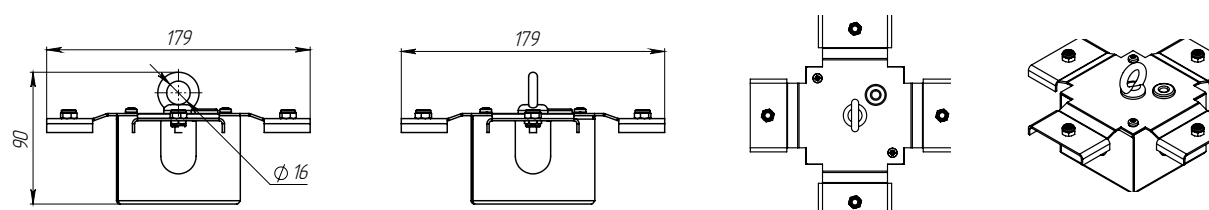
ДСО_кронштейн_109_СБ
