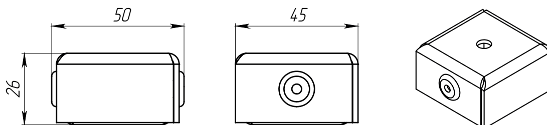
ДСО_кронштейн_СБ (антивандальный)
