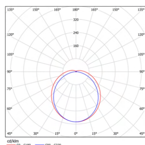
Д-косинусная
